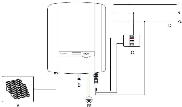
Fig. 5-1 Elektrisches Anschlussschema
