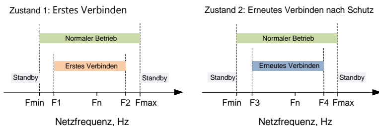
Fig. 2-8 Wechselrichterverhalten in Bezug auf die Netzfrequenz („DE“ als Beispiel)
