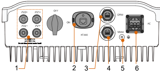
Fig. 5-2 Beschreibung der Anschlussklemmen
