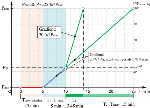
Fig. 2-10 Leistungswiederherstellung bei vorübergehender Überfrequenz (IT)
