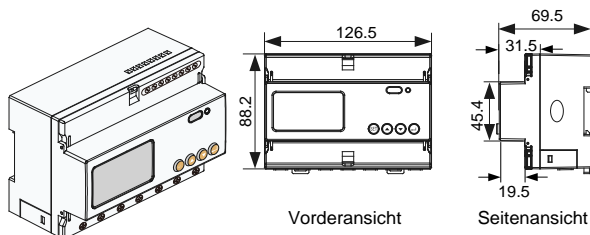
Fig. 2-6 Dreiphasiger Smart Energy Meter – Abmessungen (Einheit: mm)
