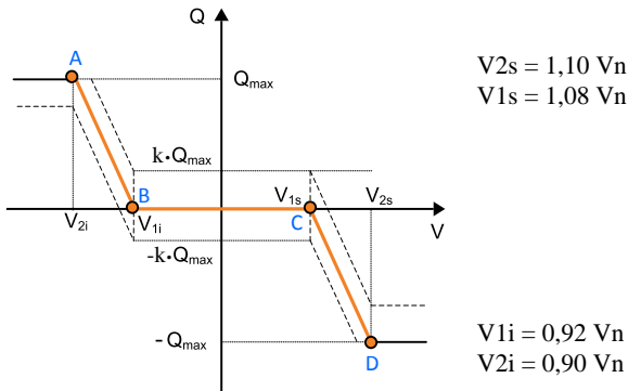
Fig. 2-13 Blindleistungs-Regulierungskurve im Q(U)-Modus für „IT“
