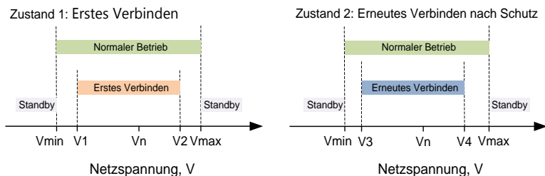
Fig. 2-7 Wechselrichterverhalten in Bezug auf die Netzspannung („DE“ als Beispiel)
