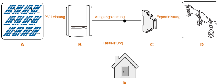
Fig. 2-1 Anwendung in einem PV-Stromsystem
