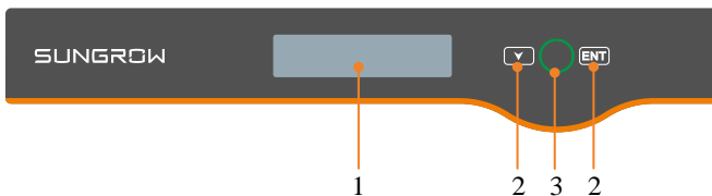
Fig. 2-4 LCD-Anzeige
