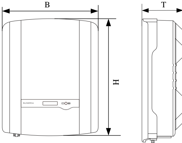
Fig. 2-3 Abmessungen des Wechselrichters
