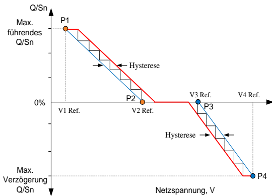
Fig. 2-12 Blindleistungs-Regulierungskurve in Q(U)-Kurve
