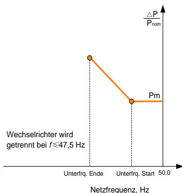
Fig. 2-11 Wirkleistungsverhalten bei Unterfrequenz
