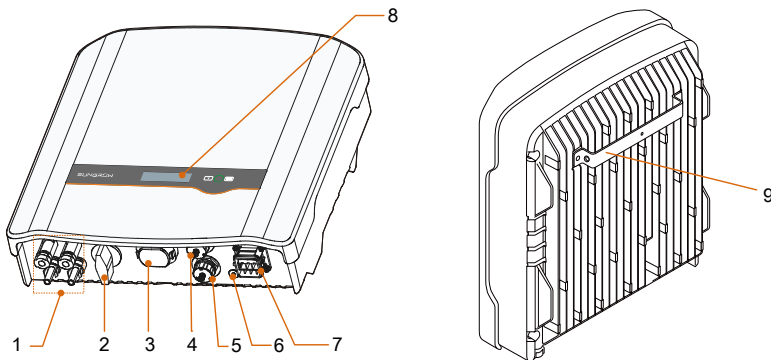
Fig. 2-2 Wechselrichteroptik (Serie -D als Orientierung)
