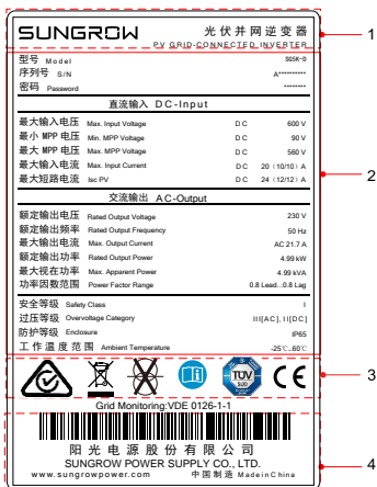
Fig. 3-2 Typenschild des Wechselrichters
