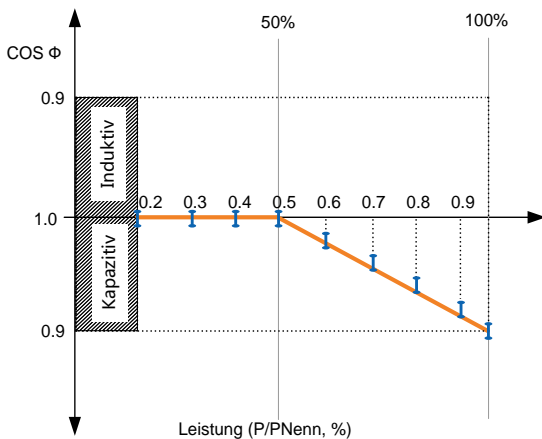
Fig. 2-14 Blindleistungs-Regelkurve im Q(P)-Modus
