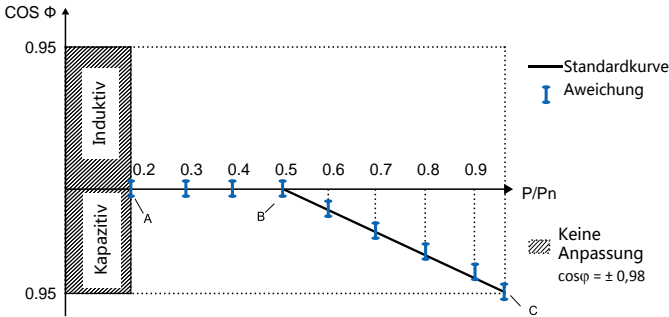
Fig. 2-15 Blindleistungs-Regelkurve im Q(P)-Modus für „IT“
