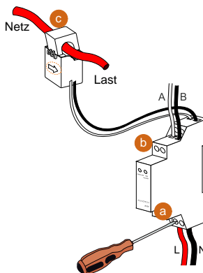
RS485 Kabel den Stromzähler
