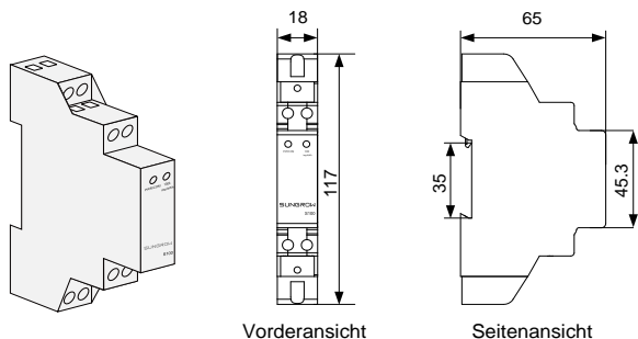
Fig. 2-5 Einphasiger Smart Energy Meter – Abmessungen (Einheit: mm)
